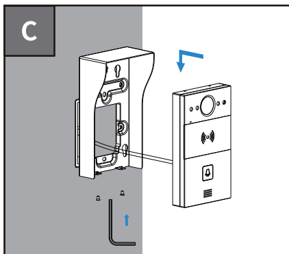
Mit Unterputzdose
